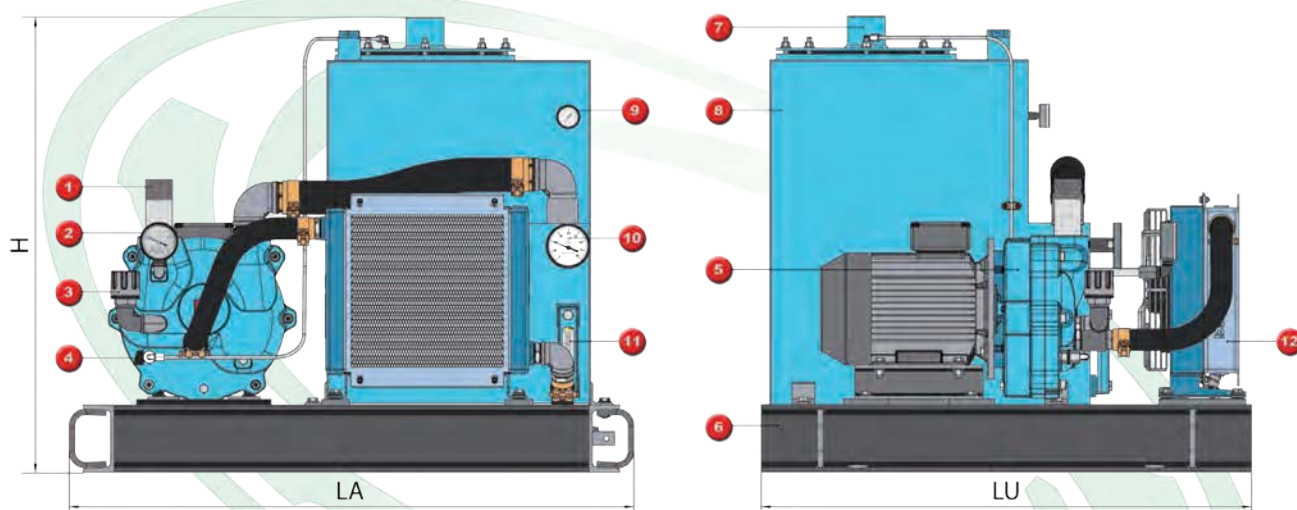
Схематичний малюнок. Розміри в (мм) з допусками до стандартів EN 735-1995. Вага в (кг), стосовно до насосів у чавуні, не сертифіковані. Schematic drawing. Dimensions in mm with tolerances to EN 735-1995 standards. Weights in Kgs, referred to pumps in cast iron, not certified.
